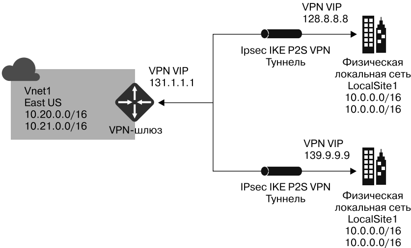
Рис. 11.30. Клиентский VPN-шлюз в Azure (источник: https://docs.microsoft.com/ru-ru/azure/vpn-gateway/vpn-gateway-about-vpngateways )
