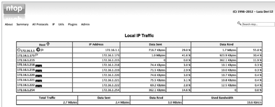
Рис. 8.9. Локальный IP-трафик в ntop
