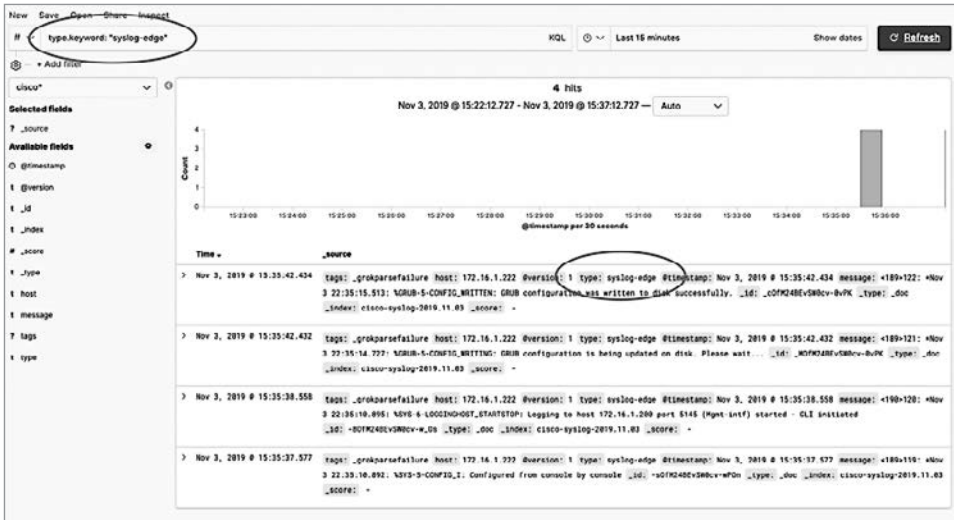
Рис. 12.11. Индекс Syslog
