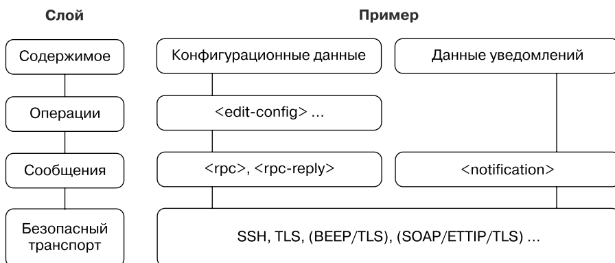
Рис. 3.5. Модель NETCONF
