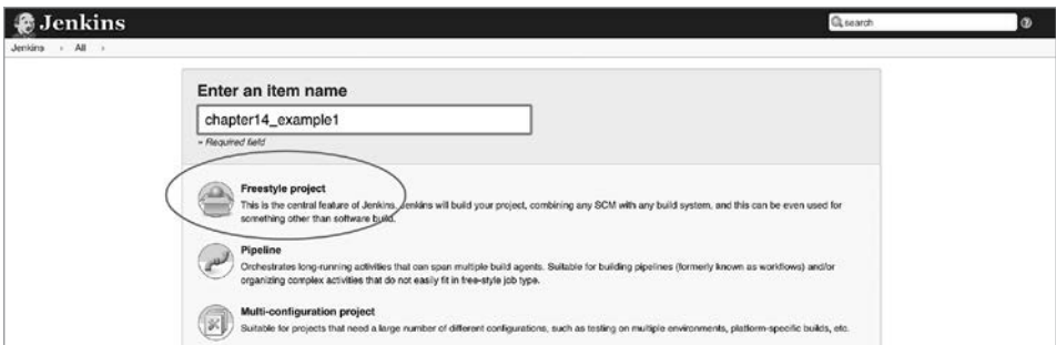
Рис. 14.5. Элемент Jenkins
