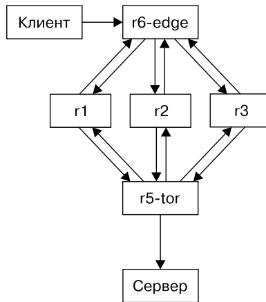
Рис. 8.7. Граф топологии 3
