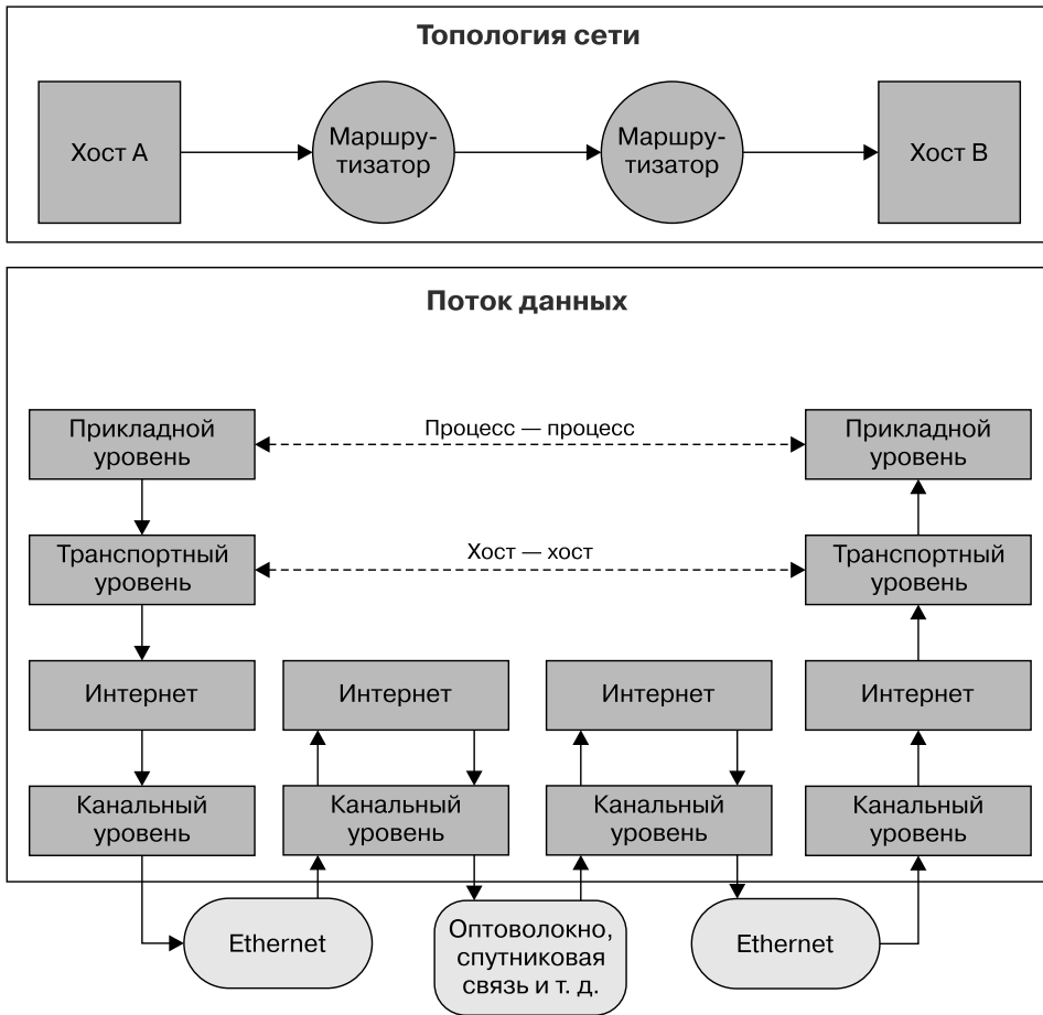
Рис. 1.5. Набор интернет-протоколов
