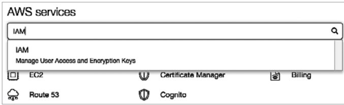
Рис. 10.3. AWS IAM
