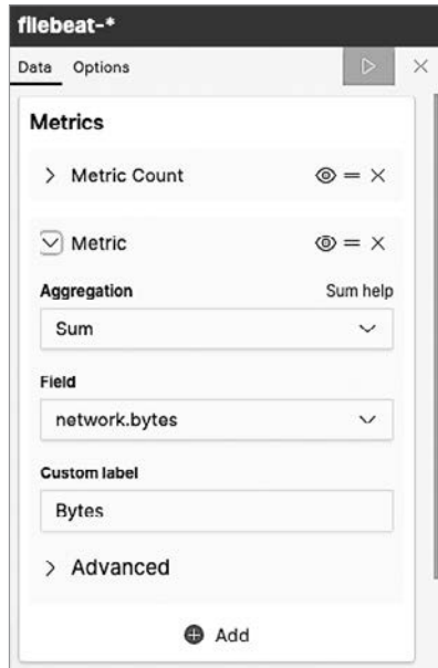
Рис. 12.30. Метрики Kibana
