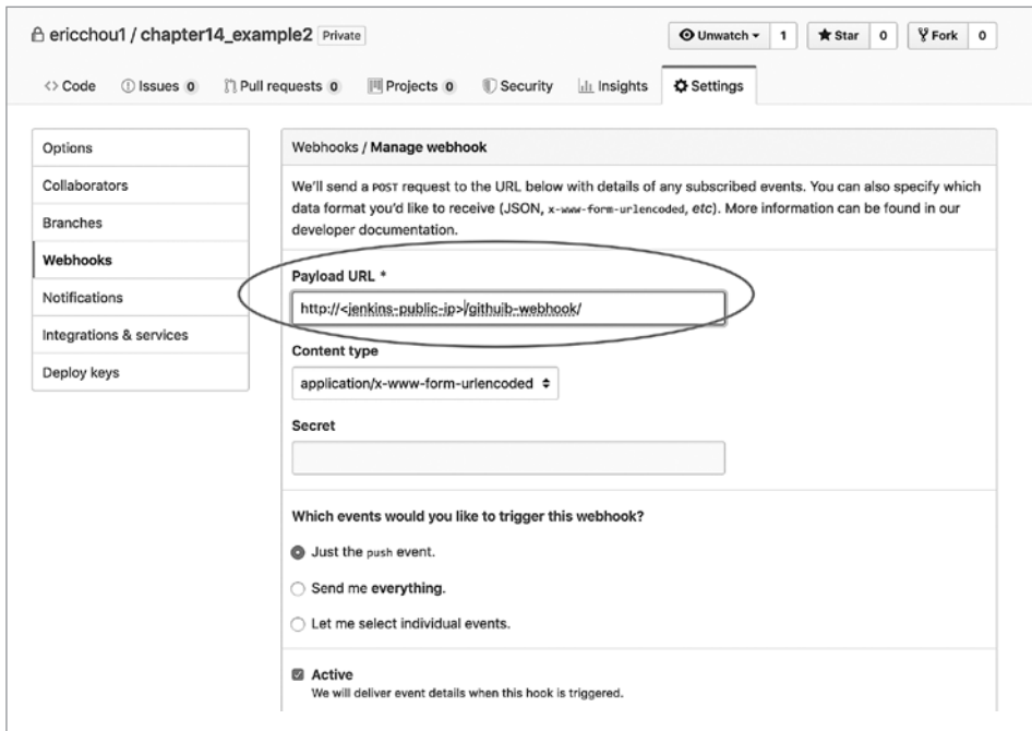
Рис. 14.26. Веб-обработчики GitHub
