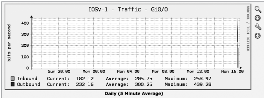
Рис. 7.15. График с усреднением за 5 минут
