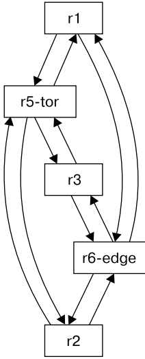
Рис. 8.5. Граф топологии 1
