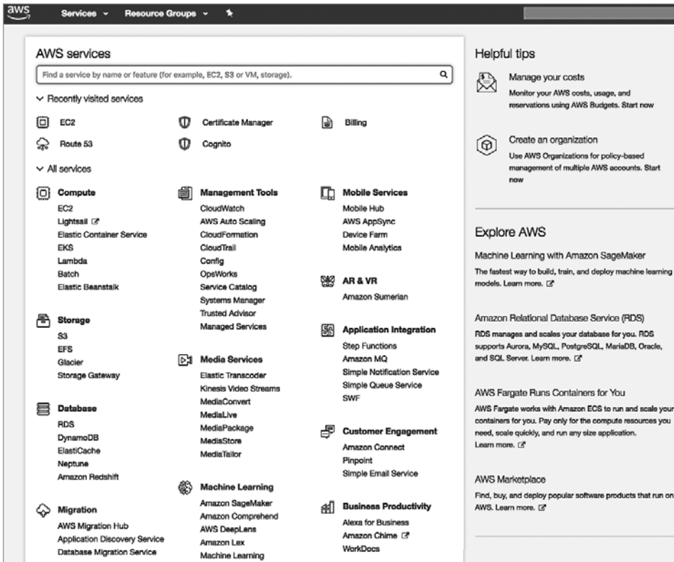
Рис. 10.2. Консоль AWS
