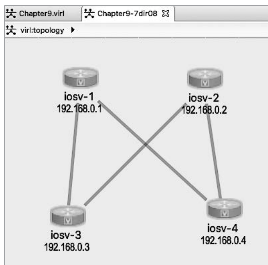
Рис. 9.2. Топология лаборатории
