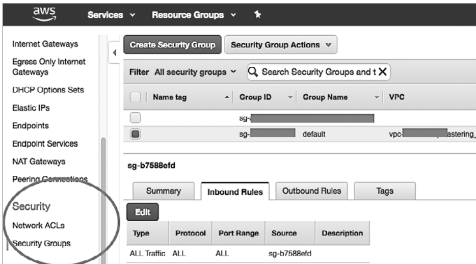
Рис. 10.21. Безопасность VPC
