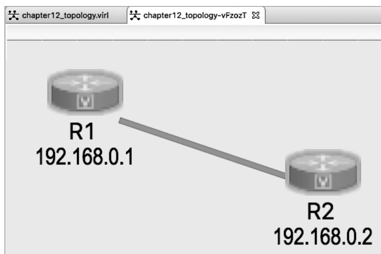
Рис. 14.4. Топология лаборатории
