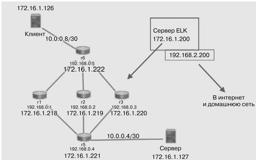
Рис. 12.2. Топология лаборатории
