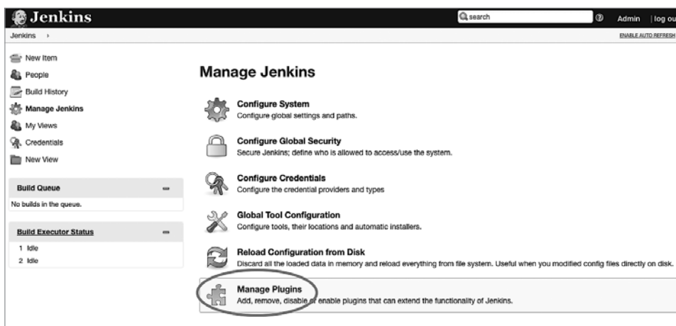
Рис. 14.14. Плагины Jenkins
