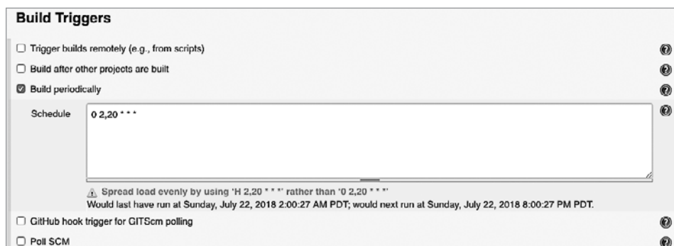
Рис. 14.10. Триггер сборки
