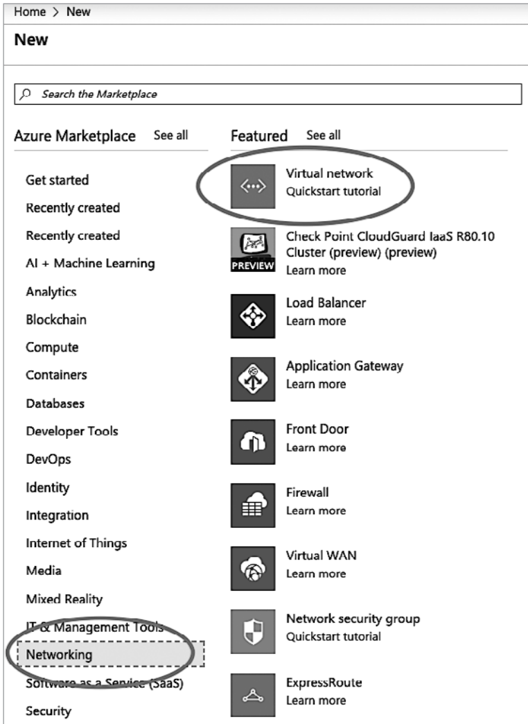
Рис. 11.12. Azure VNet
