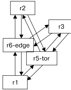
Рис. 8.6. Граф топологии 2
