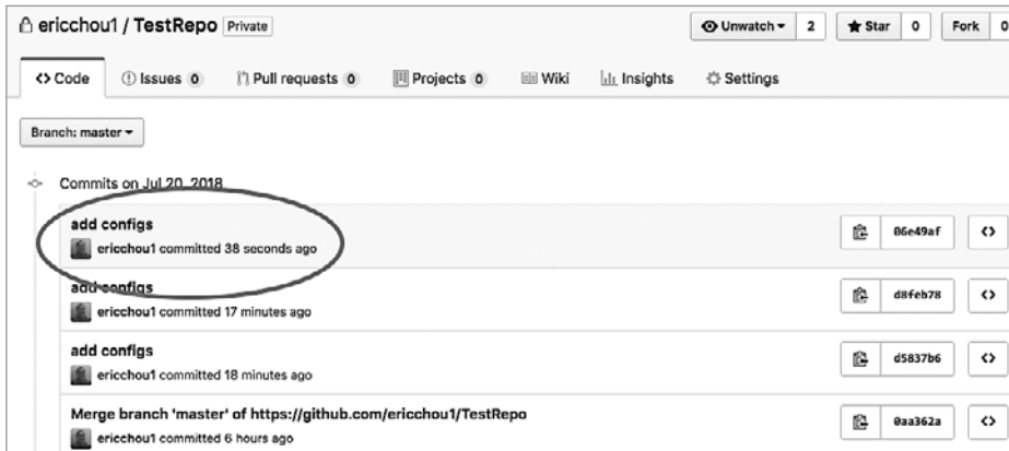
Рис. 13.13. История изменений
