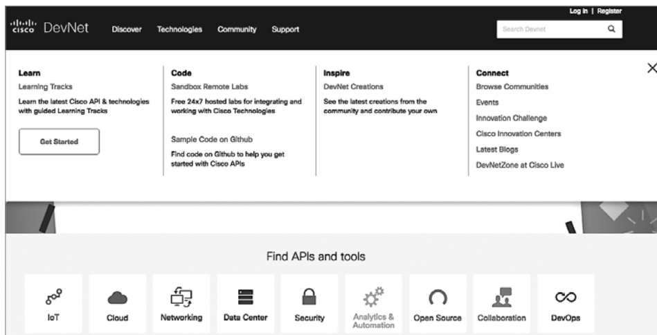
Рис. 2.6. Cisco DevNet
