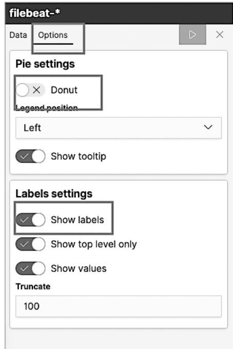
Рис. 12.26. Параметры диаграммы в Kibana
