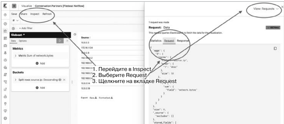
Рис. 12.20. Запрос в Kibana
