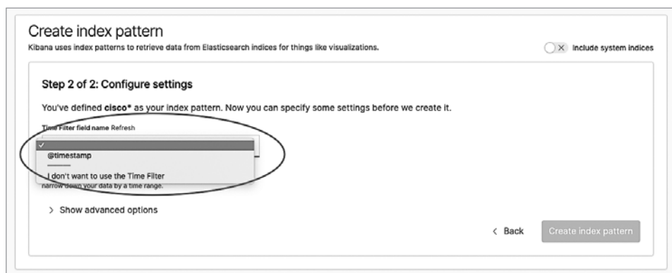
Рис. 12.9. Настройка временной метки для шаблона индекса в Elasticsearch
